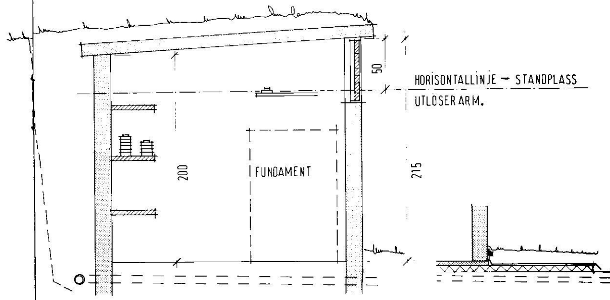
SNITT.
